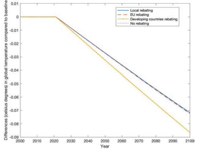
(b) \Delta global temperature (°C)
