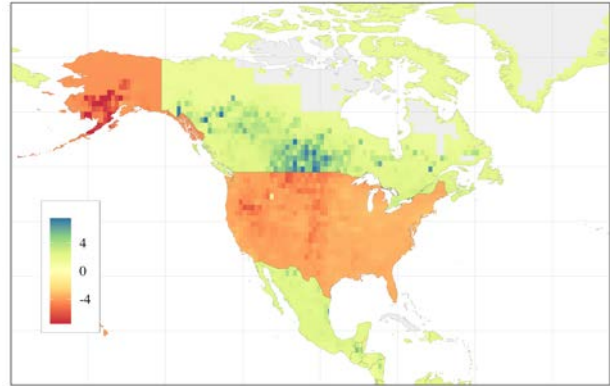
(d) % \Delta Non-agriculture, no rebating, 2100
