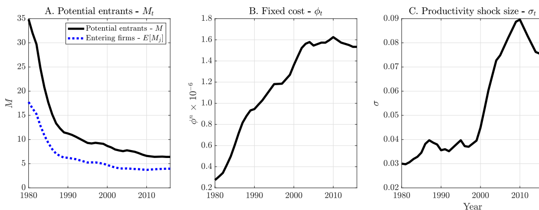
Figure 4: Parameter estimates
